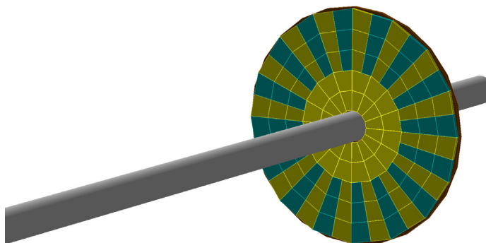
Рис. 1. Визуализация прототипа BBC в Geant4
