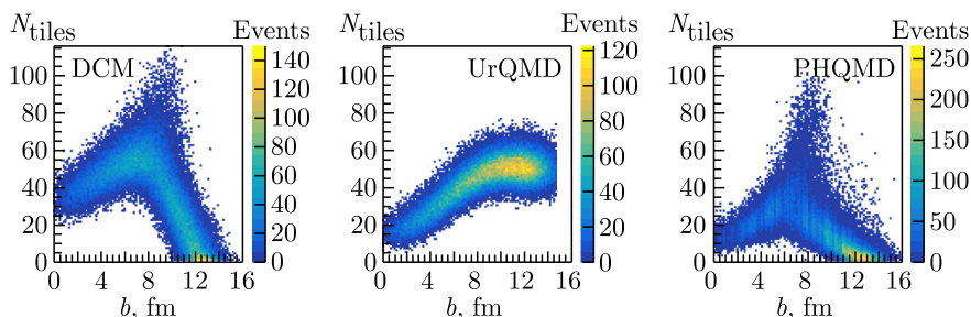
Рис. 3. Распределения зависимости множественности сработавших элементов детектора от прицельного параметра для различных генераторов событий
