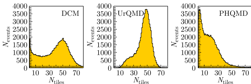
Рис. 2. Гистограммы числа сработавших элементов детектора в одном событии для различных генераторов событий
