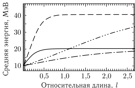
Рис. 1. Зависимость средней энергии нейтрино \langle p \rangle_l от относительной длины пробега l/l_{tp} при начальном значении \langle p \rangle_0 = 10 МэВ и температурах T = 5 МэВ (сплошная и штрихпунктирная линии) и T = 10 МэВ (штриховая и штрихпунктирная с тремя точками линиями). Влияние эффекта переноса энергии показано штрихпунктирной и штрихпунктирной с тремя точками линиями, тогда как сплошная и штриховая линии соответствуют результатам с учетом диффузионного члена для распределения Максвелла–Больцмана
