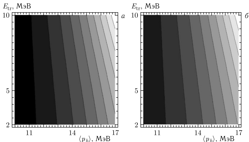
Рис. 3. Зависимость относительной скорости счета (см. (12)) от пороговой энергии при средних энергиях нейтрино электронного аромата \langle p \rangle_e = 10 МэВ и тяжелой-лептонной компоненты \langle p \rangle_h , изменяющейся от 10 до 17 МэВ: а) нормальный порядок масс; б) обратный порядок масс. Контуры представляют изолинии постоянного значения R_{\text{SN}}(E_{\text{th}})/R_0 (см. текст) с равномерным шагом в интервале от 1 до 5 (а) и 10,5 (б) для нормального и обратного порядка масс соответственно
