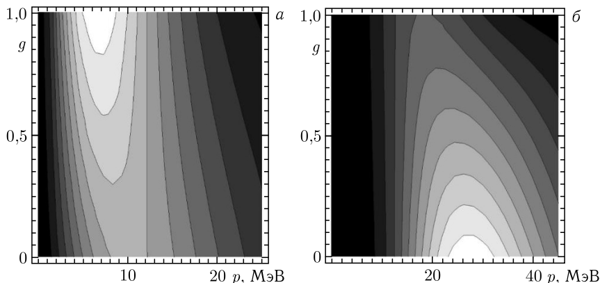
Рис. 2. Энергетическая зависимость потока нейтрино (а) и скорости счета (см. (11)) (б) в зависимости от значения параметра смешивания ароматов g при средних энергиях тяжелолептонных \langle p \rangle_h = 15 МэВ и электронных \langle p \rangle_e = 10 МэВ компонент нейтрино. Границы серых областей соответствуют изолиниям постоянных величин (в произвольных единицах) с равномерным шагом в интервале от 0 до 0,08 для спектра и до 1300 для сигнальных событий
